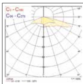
4.000K Asimmetrico
