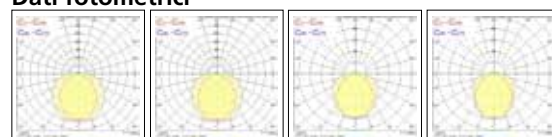
1,265mm - Versione Single - 23W 1,565mm - Versione Single - 37W 1,265 mm - Versione Twin 44W 1,565mm - Versione Twin - 75W Curve fotometriche delle versioni 662mm Single e Twin disponibili su richiesta o sul sito web
