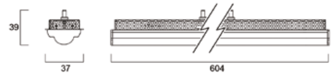
Tide Symmetrisch/Dubbel Asymmetrisch Inbouwversie
