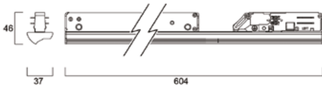
Tide Asymmetrisch Railversie
