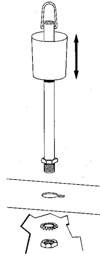
SUSPENSION A 2 TIGES INDÉPENDANTES DS2
